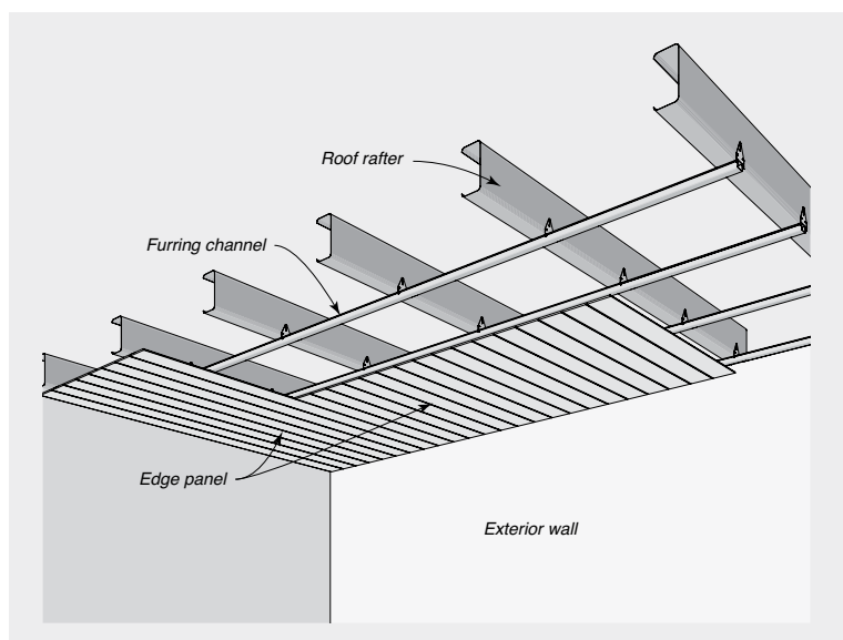
FIGURE 2.04 Edge Cladding
